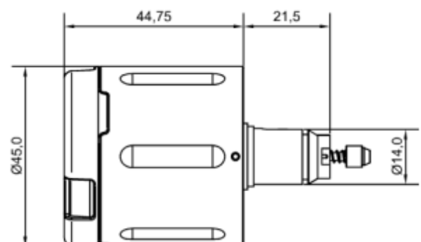
IK CX6180 für Außentüren (IP 66)
